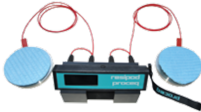
Комплект для измерения объемного сопротивления
